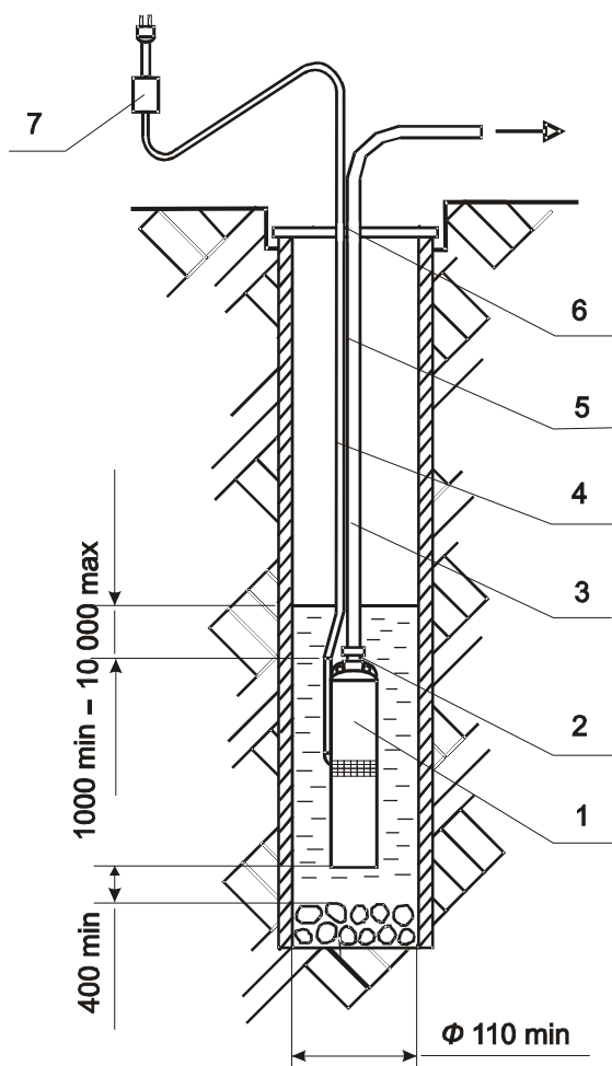
Рис 4. Схема установки электронасоса БЦПЭ в скважину (размеры в мм). 1 - электронасос; 2 - хомут трубопровода; 3 - трубопровод; 4 - шнур сетового питания; 5 - трос; 6 - место крепления подвески; 7 - коробка конденсаторная.
