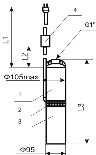
Рис. 1 Габаритные и присоединительные размеры
