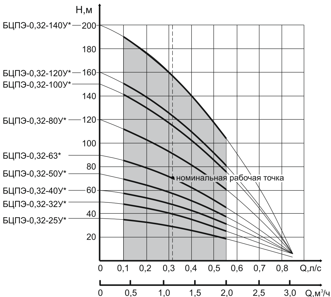
Рис. 2 Напорные характеристики электронасосов H - напор в метрах водного столба, Q - объемная подача. ■ - оптимальная зона эксплуатации электронасосов
