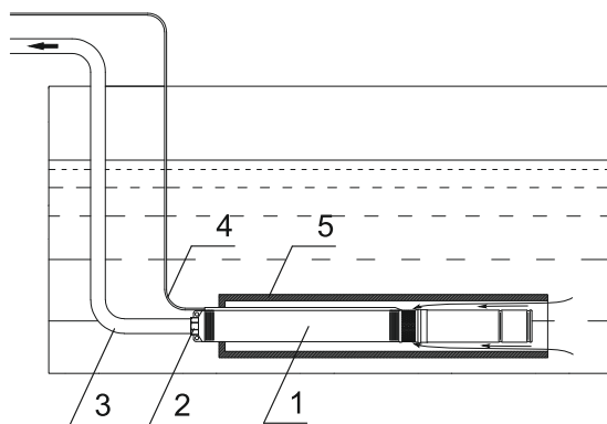
Рис 4. Схема установки электронасоса БЦПЭ в скважину (размеры в мм). 1 - электронасос; 2 - хомут трубопровода; 3 - трубопровод; 4 - шнур сетового питания; 5 - трос; 6 - место крепления подвески; 7 - коробка конденсаторная.
